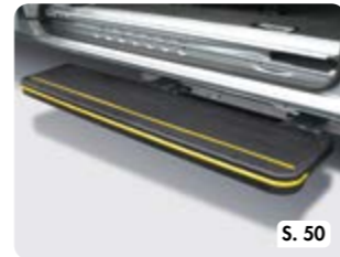
S. 50 Serie SCE | Seitliche Heavy-Duty elektrische Schwenk-Trittsstufe
